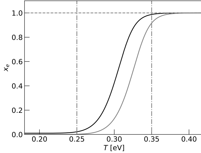
Figura 26 : Evoluzione della frazione di elettroni liberi durante la ricombinazione con le correzioni per le approssimazioni.
